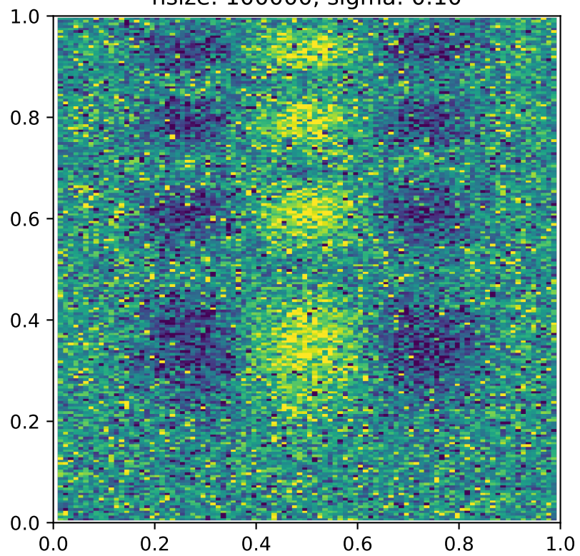
nsize: 100000, sigma: 0.10
