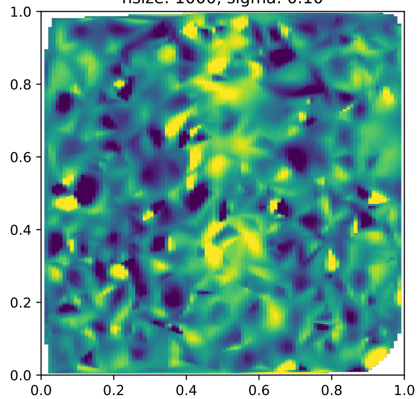
nsize: 1000, sigma: 0.10
