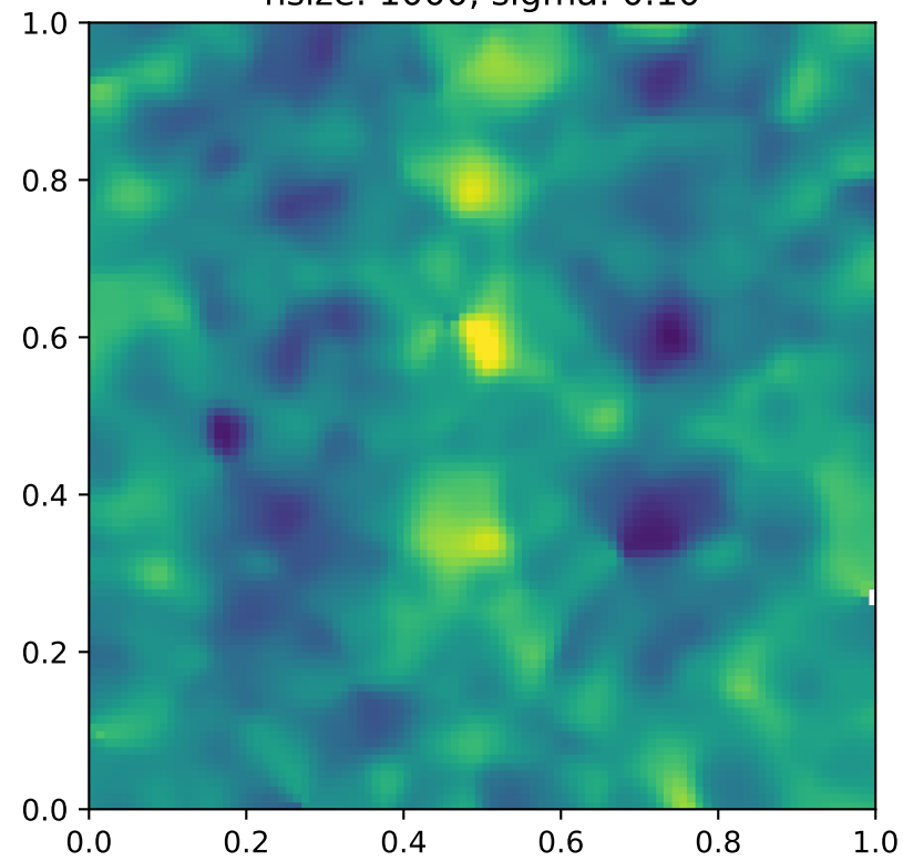
nsize: 1000, sigma: 0.10
