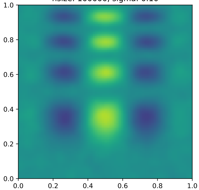
nsize: 100000, sigma: 0.10
