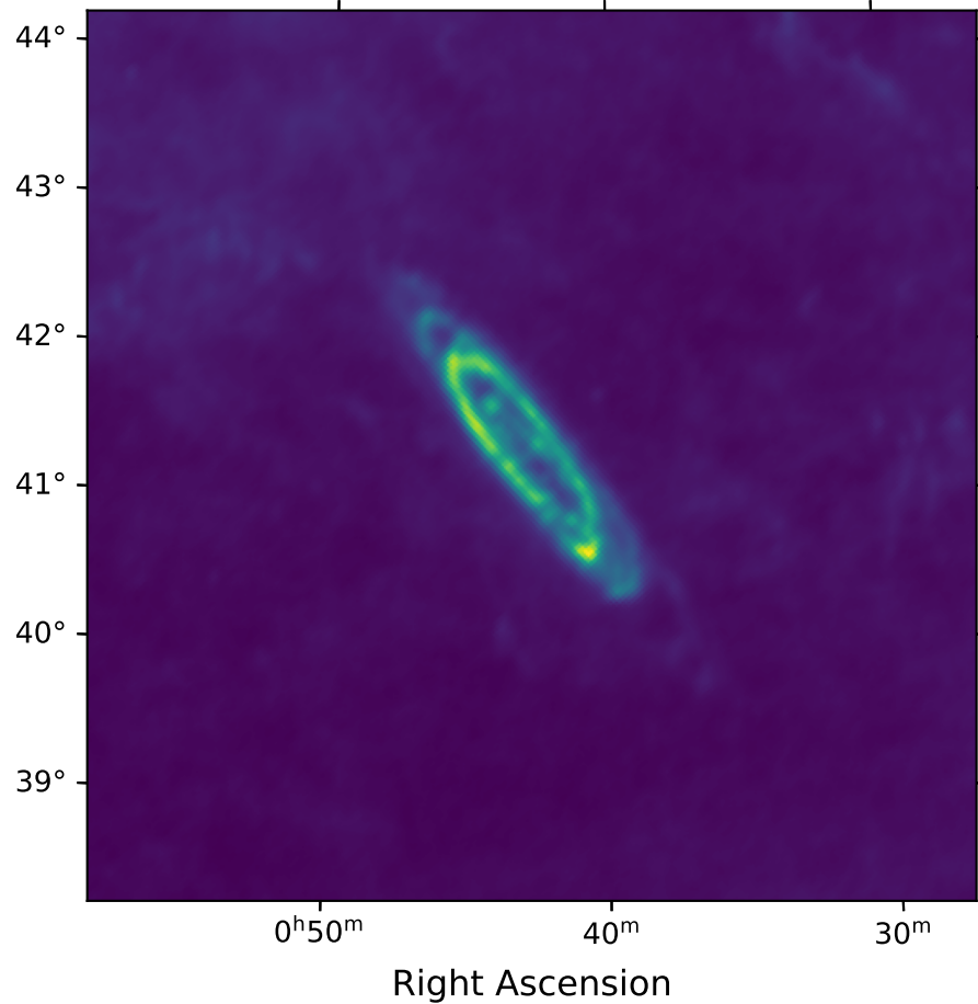
Planck 857 GHz
